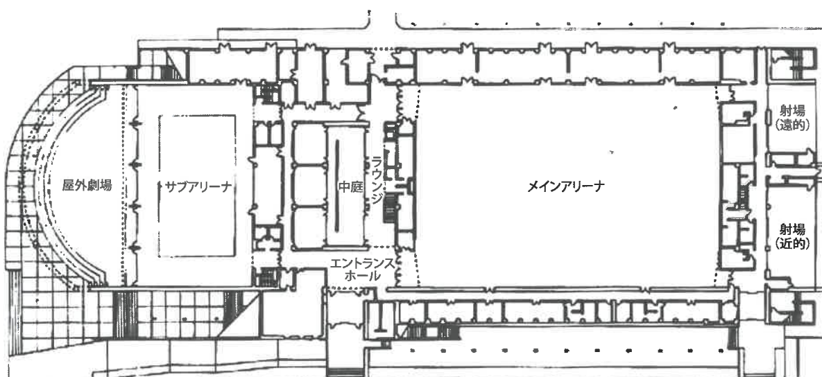
1 階平面図
